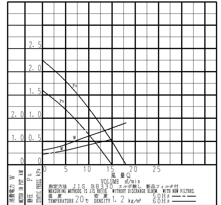
性能曲線図 PERFORMANCE CURVE
